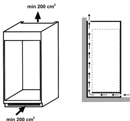
Рисунок Б.4 - Схема циркуляции воздуха вокруг холодильного прибора Рисунок Б.4 - Схема циркуляції повітря навколо холодильного приладу Сурет Б.4 - Тоңазытқыш прибор айналасындағы ауа айналысының схемасы
